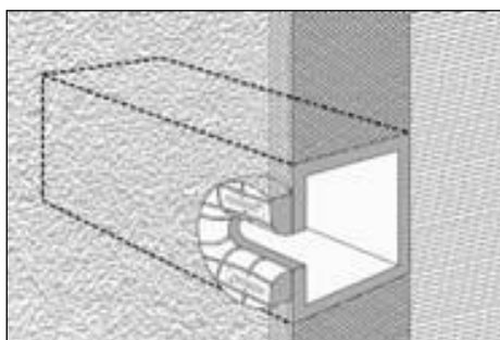
Schematický náčrtek téže budky, instalované ve vrstvě zateplení v atikovém prostoru objektu v místě stávajících VO
